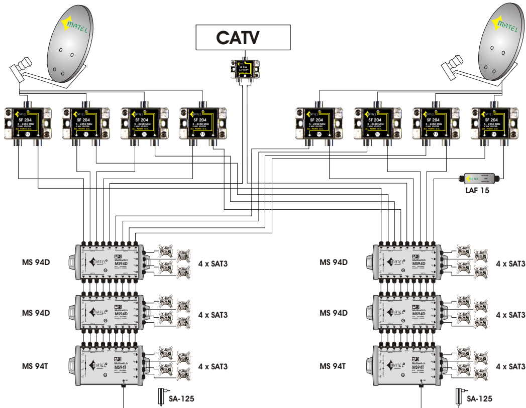
Συνδεσμολογία διακλαδωτών, σε ομαδική δορυφορική εγκατάσταση 24 παροχών.
